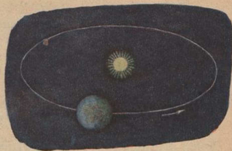
Движение земли вокруг солнца
